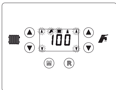
рис. 17 - Режим TEST (мощность системы отопления= 100%)
