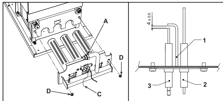
рис. 21 - Очистка блоков горелок и электродов
