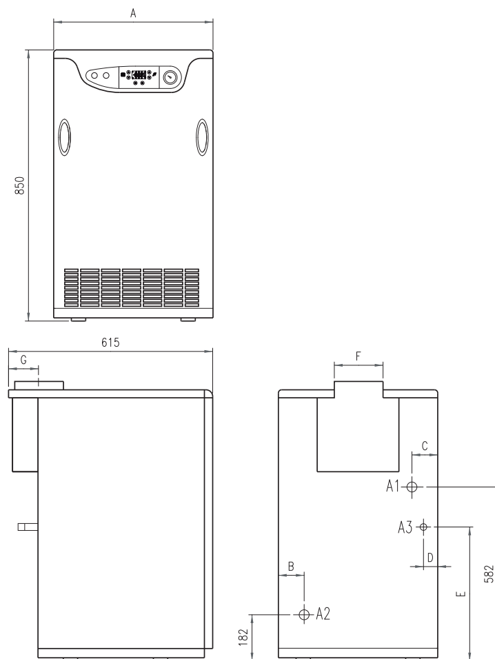
рис. 22 - Габаритные размеры и присоединения
