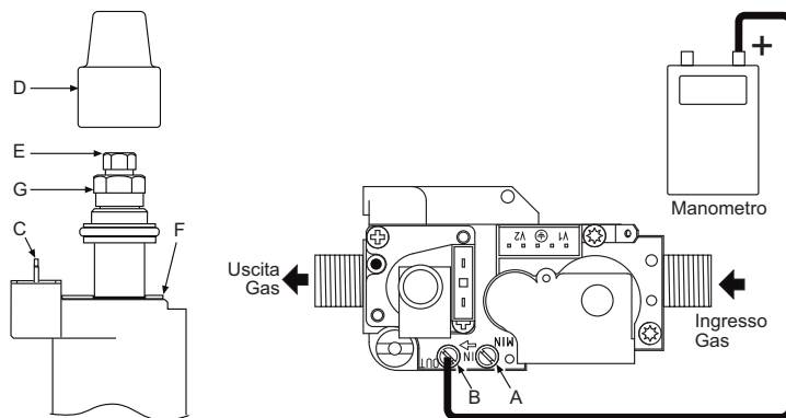
рис. 18 - Газовый клапан
