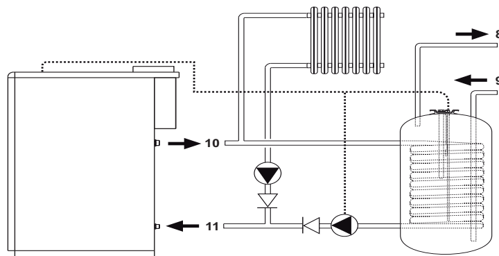
рис. 16 - Схема соединений с внешним бойлером
