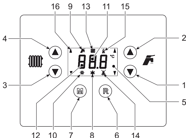
рис. 1 - Панель управления
