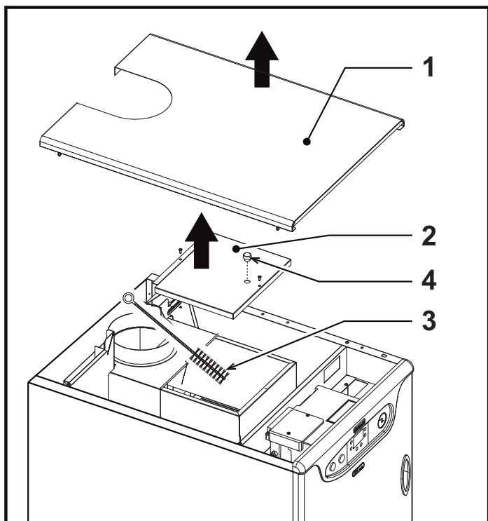
рис. 19 - Очистка котла
