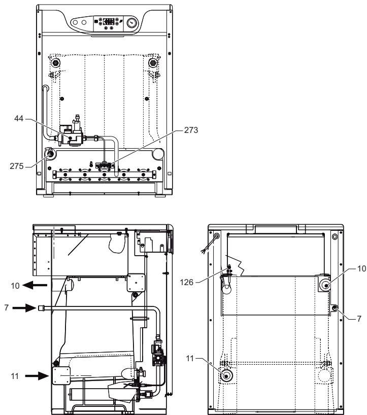
рис. 23 - Основные узлы
